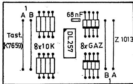
Bestückungsplan
