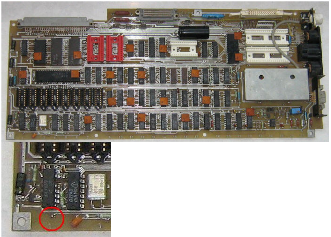
Z9001, Serie 84. Das einfachste Unterscheidungsmerkmal zur Serie 85 ist der fehlende Kondensator links unten an der Markierungsstelle 1. Die Serie 85 hat hier zwei Durchkontaktierungen, in denen ein zweiter Kondensator steckt.
