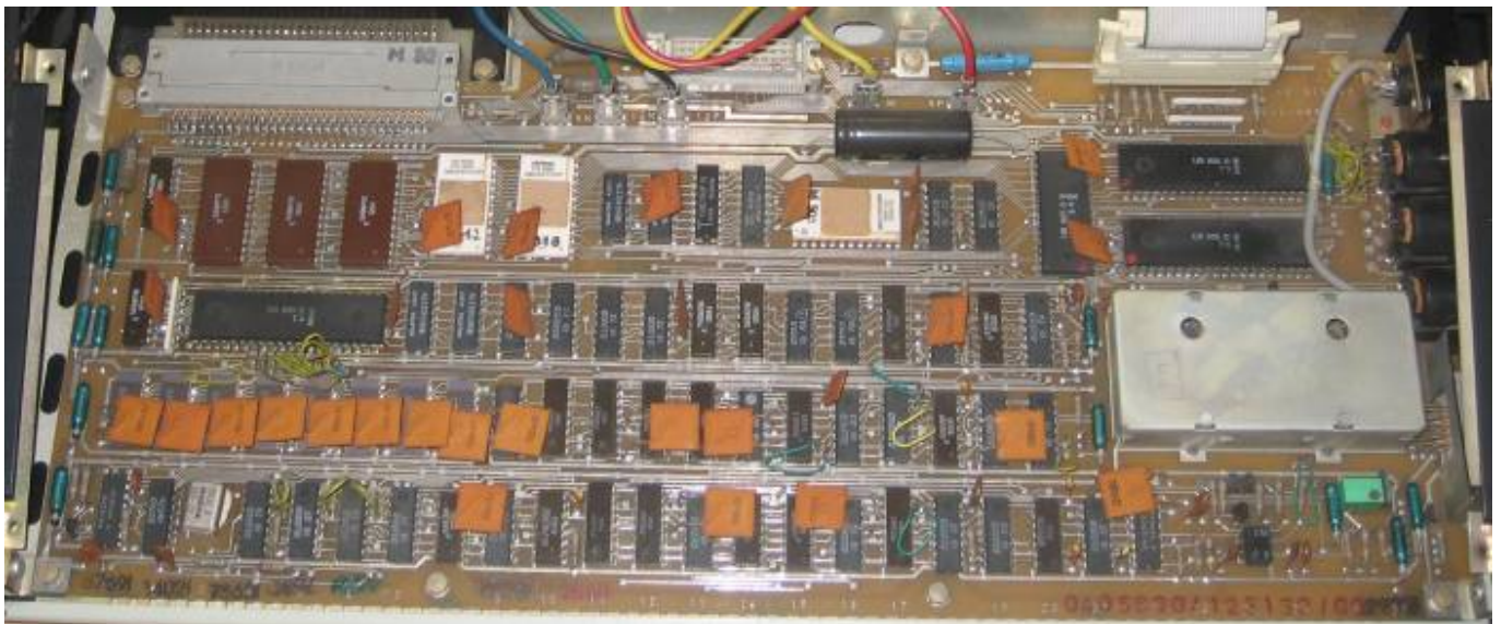
Z9001, Serie 85. Man erkennt unten links zwei Kondensatoren. Oben sind die SYSTEM-EPROMS M512 und M513 zu erkennen, rechts befindet der Zeichensatz-EPROM M505.
