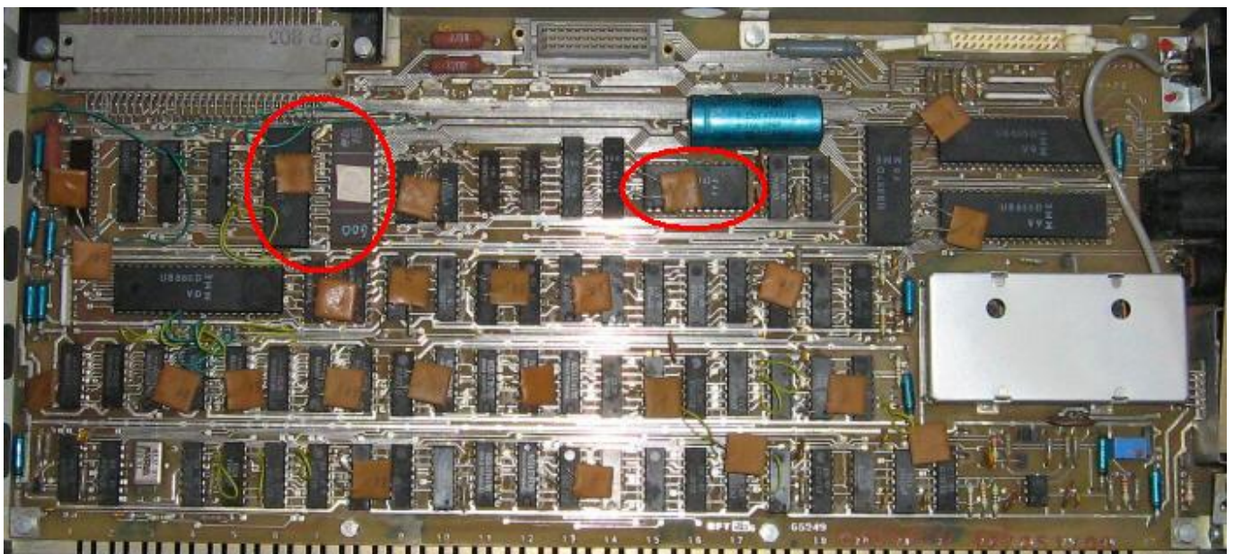
KC87.21. Deutlich sind links oben die großen (E)PROMs 600 und 608 anstelle der 5 größeren
