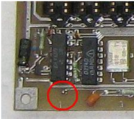
Z9001, Serie 84. Das einfachste Unterscheidungsmerkmal zur Serie 85 ist der fehlende Kondensator links unten an der Markierungsstelle 1. Die Serie 85 hat hier zwei Durchkontaktierungen mit einem Kondensator.
