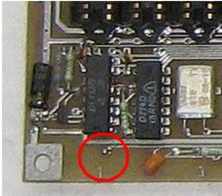
Z9001, Serie 84. Das einfachste Unterscheidungsmerkmal zur Serie 85 ist der fehlende Kondensator links unten an der Markierungsstelle 1. Die Serie 85 hat hier zwei Durchkontaktierungen mit einem Kondensator.
