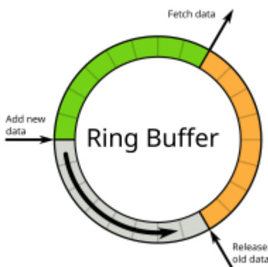
Bild: https://de.wiktionary.org/wiki/Ringpuffer
