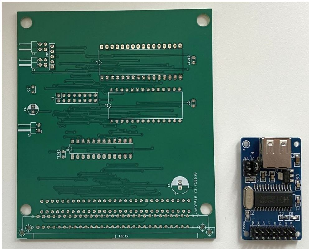
einfaches Modul,nur CH376-Aufsatz, Platine von „felge“, und das benötigte USB-CH376-Modul
