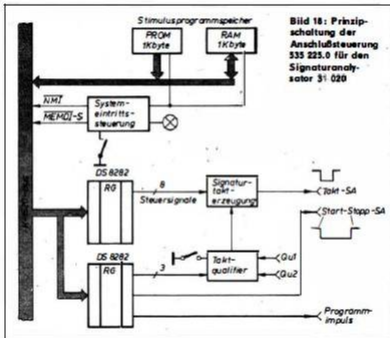
Anschluss Signaturanalysator an ASA, aus der Reparaturanleitung des Z9001; Bild 18
