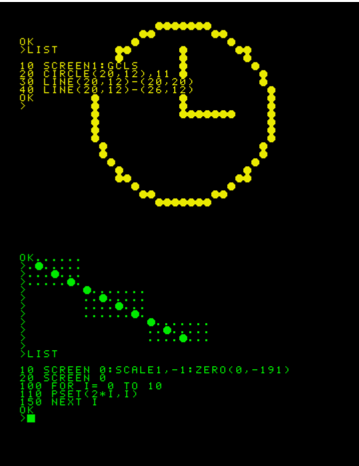
Grafik-Treiber GRAF11 für Testauflösung 40×24 „Pixel“. Im Download-Paket ist auch eine angepasste Version des Uhrenprogramms UHR11.; Weiteres Beispiel mit einer frühen Testversion. Die kleinen Punkte sind 'gelöschte' Pixel bei einer Ansteuerung wie beim originalen Grafikzusatz; es wurden also
