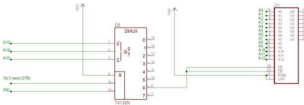
Anpassung des Adressdecoders auf dem FDC Modul und Installation eines Bootroms (U2764) auf der Adresse C000-C7FF
