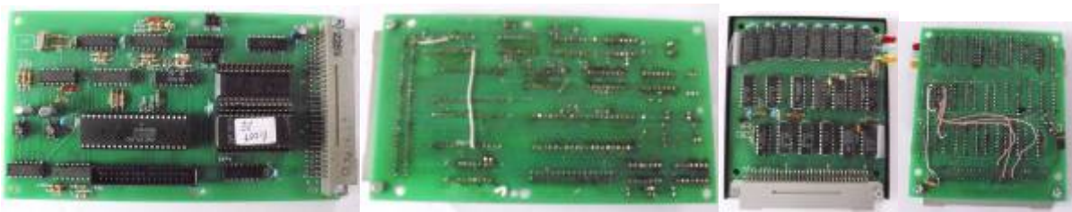
umgebautes BIC-Floppy-Modul mit BOOT-ROM, umgebautes 64K-RAM-Modul
