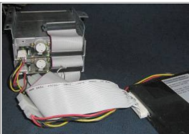
Die Laufwerke stecken in einem Floppyrahmen aus einem alten PC. Das obere Laufwerk ist A, darunter B. Anstelle des 3.5,-A kann ich an den Steckverbinder auch mein 800K-5 1/4“-Laufwerk anschließen.
