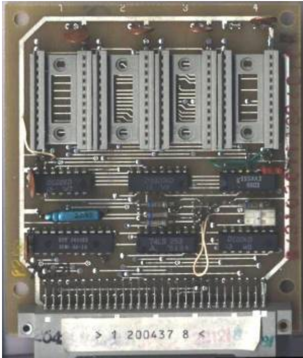
Z1013-ROM-Modul
