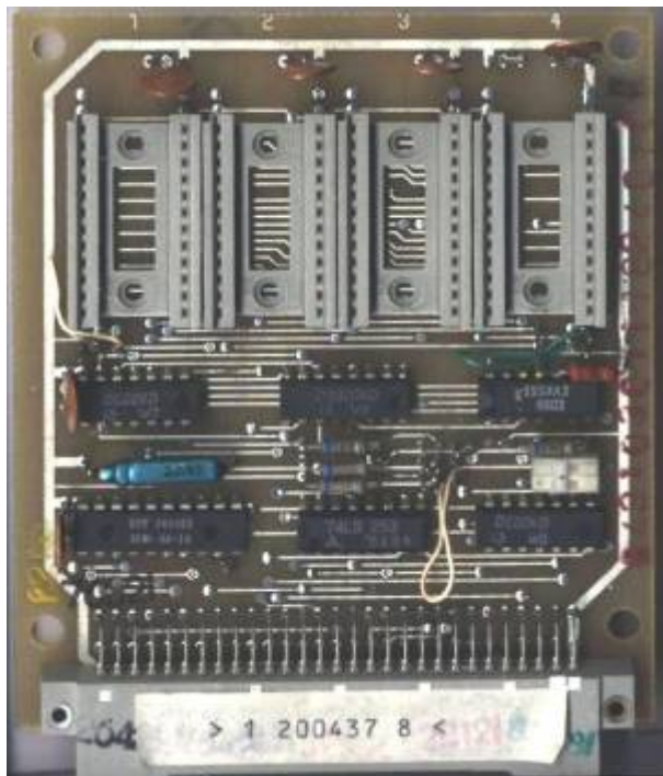
Z1013-ROM-Modul
