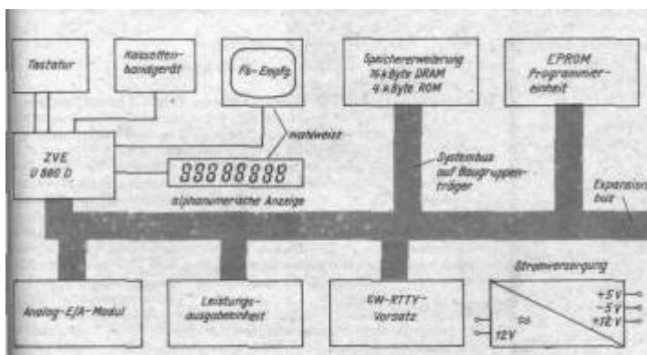
Bild 2. Darstellung des Mikrorechner-Bausatzes mit den gegenwärtig vorgesehenen Erweiterungen
