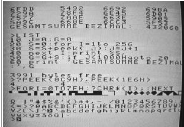
Das System 3.2 von Frank Prüfer in Aktion. Oben die Prüfsummen, darunter das Programm, dann Anzeige des Zeichensatzes.
