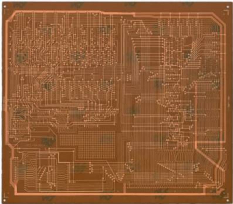
AC1 (Titelseite FA 12/83), Leiterplatte Fotomontage LS+BS (zweiseitig, nichtdurchkontaktiert, 250 mm x 300 mm !)
